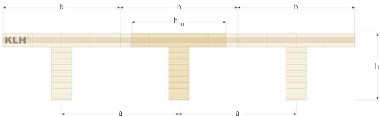
Abb. 5: Abmessungen des Plattenbalkenquerschnitts
